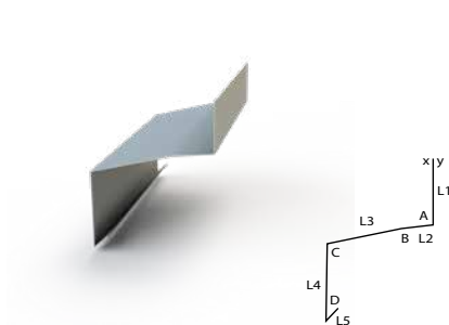
Tropfprofil 2
