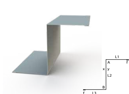
Z-Profil
