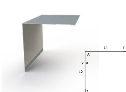
Außeneckprofil
