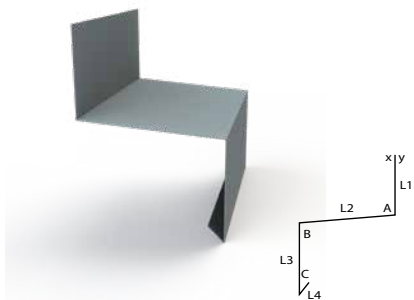
Tropfprofil
