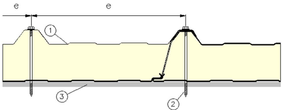
Dachelement "SAB D-TL" Befestigung am Obergurt
